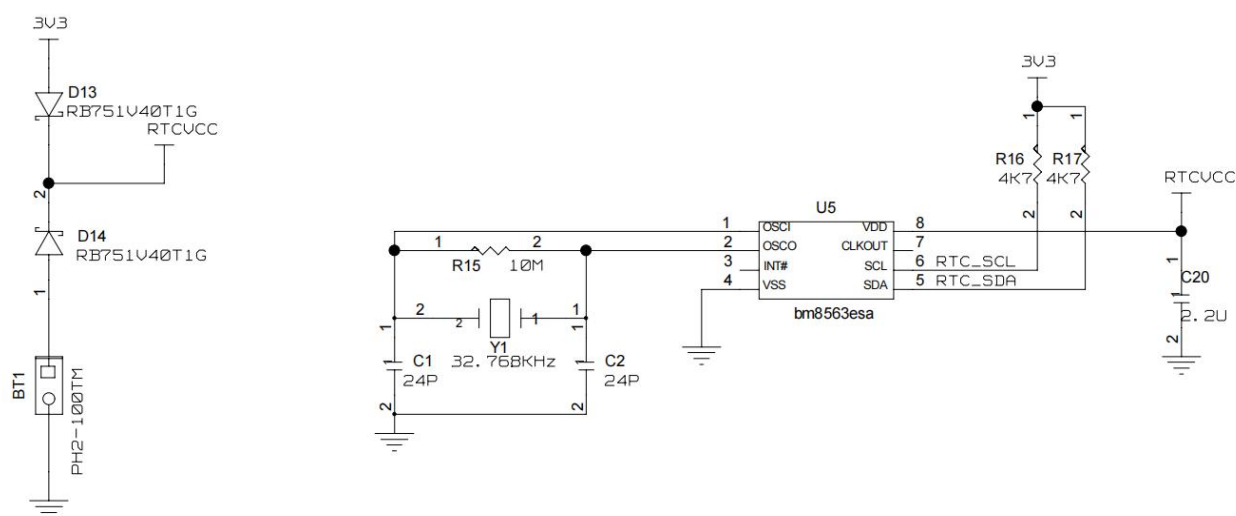
RTC 电路
