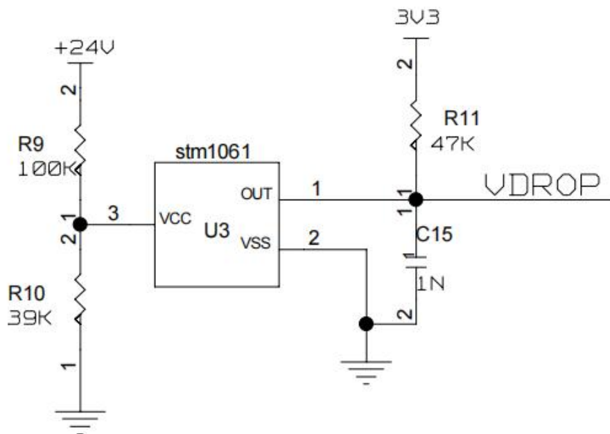
掉电保存电路
