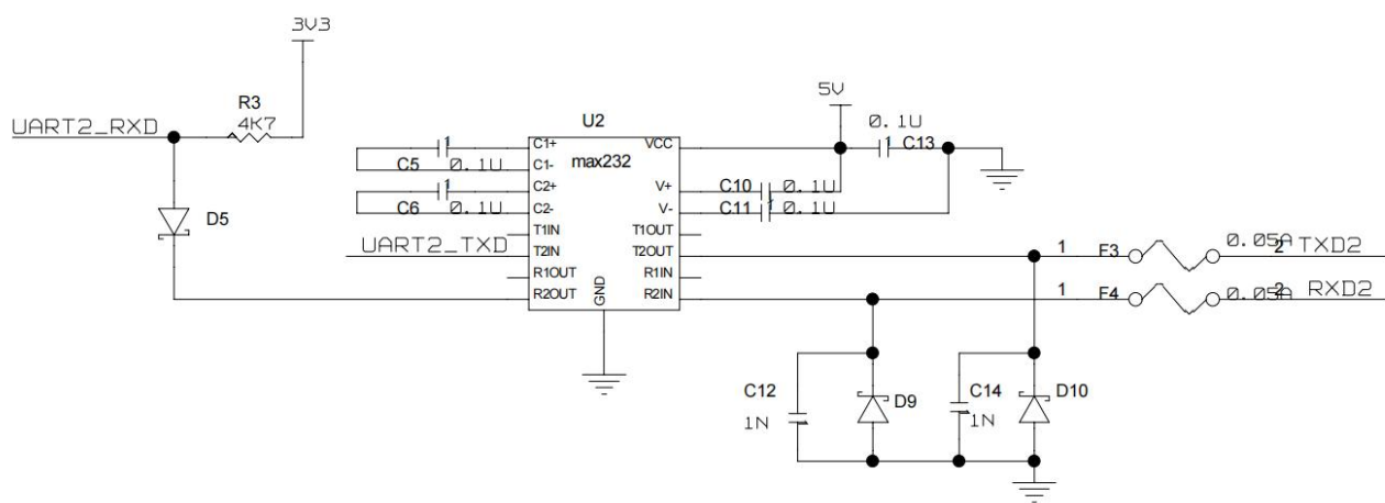
RS232参考电路
