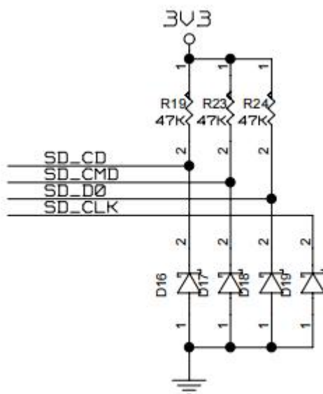
SD 卡参考电路
